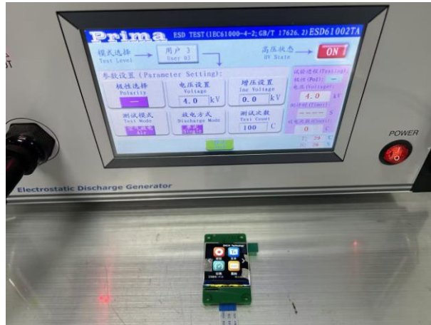
图 4-2 ESD 测试图
