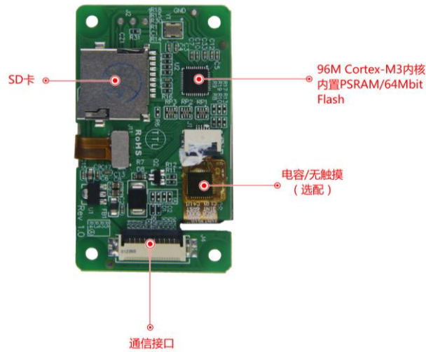
图 1-3 硬件配置图
