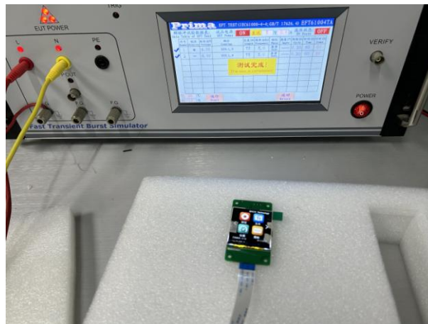
图 4-4 EFT 测试图
